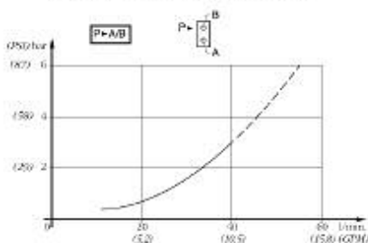
P→A/B TEMPERATURA OLIO 50°C - VISCOSITÀ 15cP
