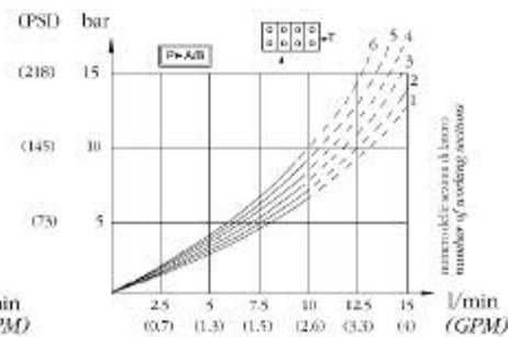
A/B<T- TEMPERATURA OLIO 50°C - VISCOSITÀ 3,5 cP
