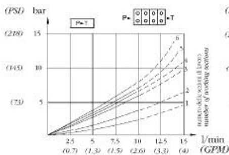
P<T- TEMPERATURA OLIO 50°C - VISCOSITÀ 3,5 cP
