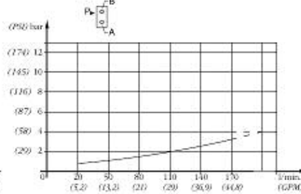
PV/B - TEMPERATURA OLIO 50°C - VISCOSITÀ 3,5'E
