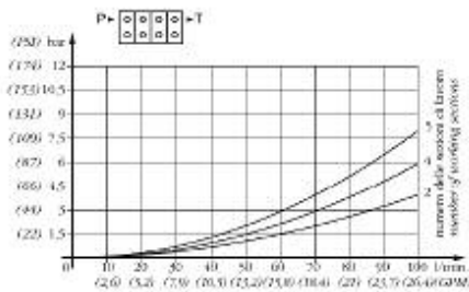
1P1 - TEMPERATURA OLIO 50°C - VISCOSITÀ 3,5P
