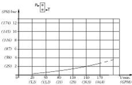
2T - TEMPERATURA OLIO 50°C - VISCOSITÀ 3,5'E
