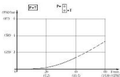
P→T TEMPERATURA OLIO 50°C - VISCOSITÀ 15cP
