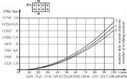
1P2/B - TEMPERATURA OLIO 50°C - VISCOSITÀ 3,5P
