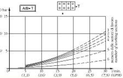
A/B/T - TEMPERATURA OLIO 50°C - VISCOSITÀ 3,5cP
