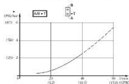
A/B→T TEMPERATURA OLIO 50°C - VISCOSITÀ 15cP
