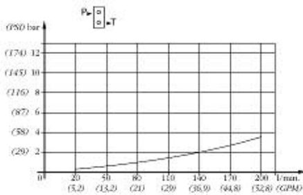
PA/T - TEMPERATURA OLIO 50°C - VISCOSITÀ 3,5'E
