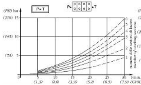
1/T - TEMPERATURA OLIO 50°C - VISCOSITÀ 3,5cP
