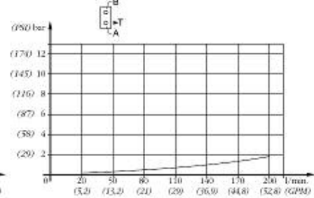
A/TPT - TEMPERATURA OLIO 50°C - VISCOSITÀ 3,5'E
