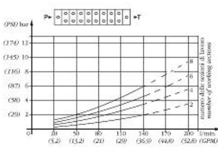
PT - TEMPERATURA OLIO 50°C - VISCOSITÀ 3,5'E
