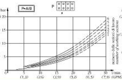
1/A/B - TEMPERATURA OLIO 50°C - VISCOSITÀ 3,5cP
