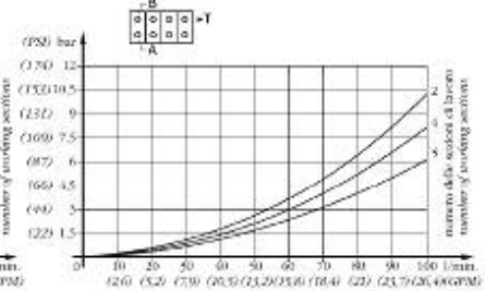
A1P1 - TEMPERATURA OLIO 50°C - VISCOSITÀ 3,5P
